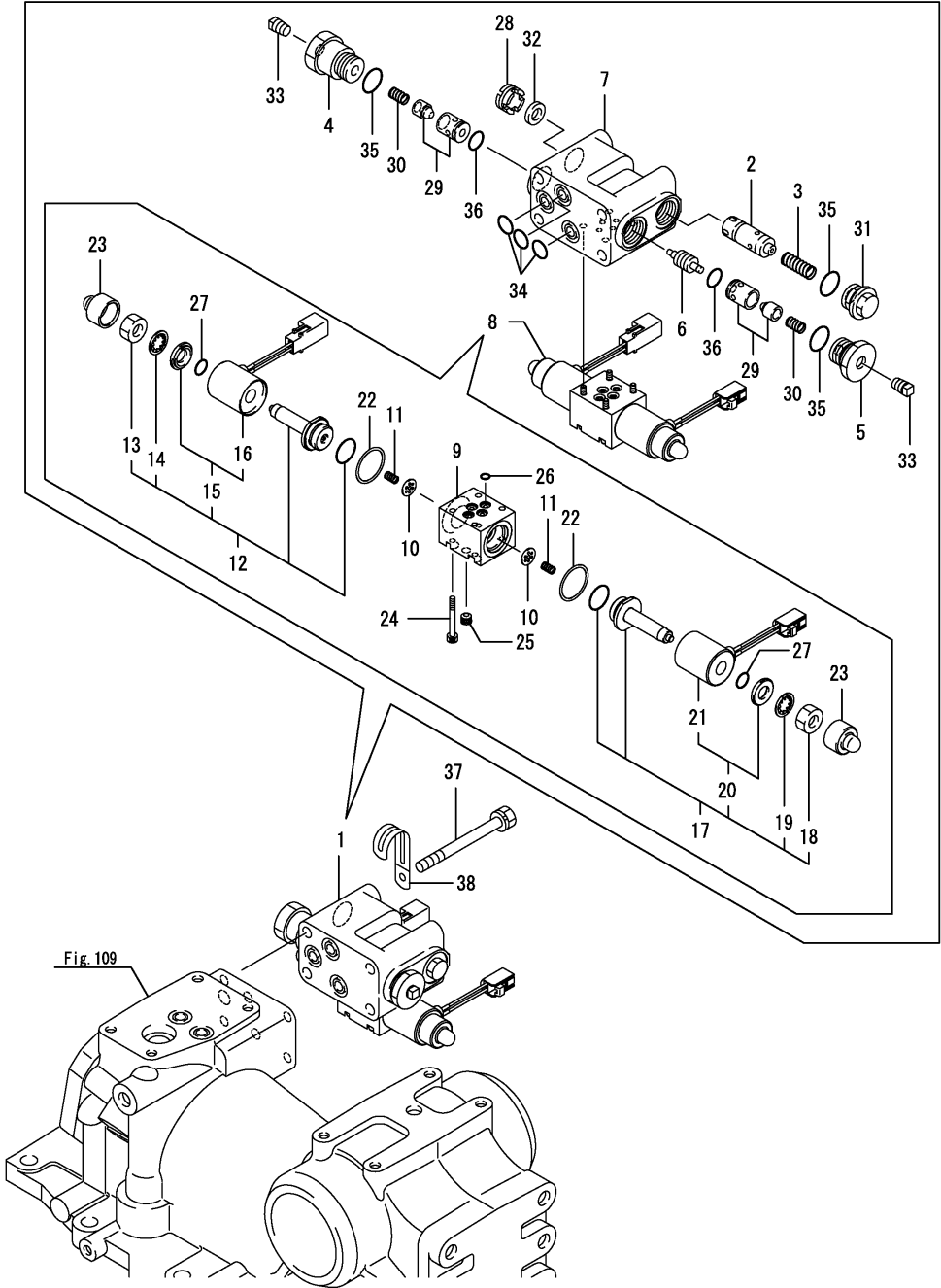
Fig.169. 수평 제어
