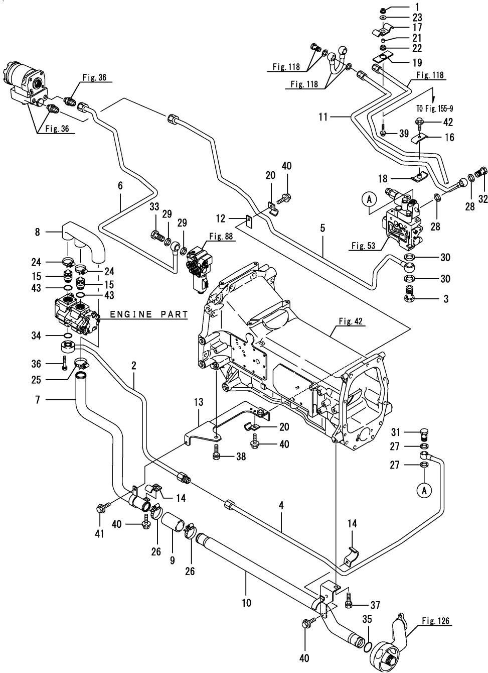
Fig.124. 유압배관
