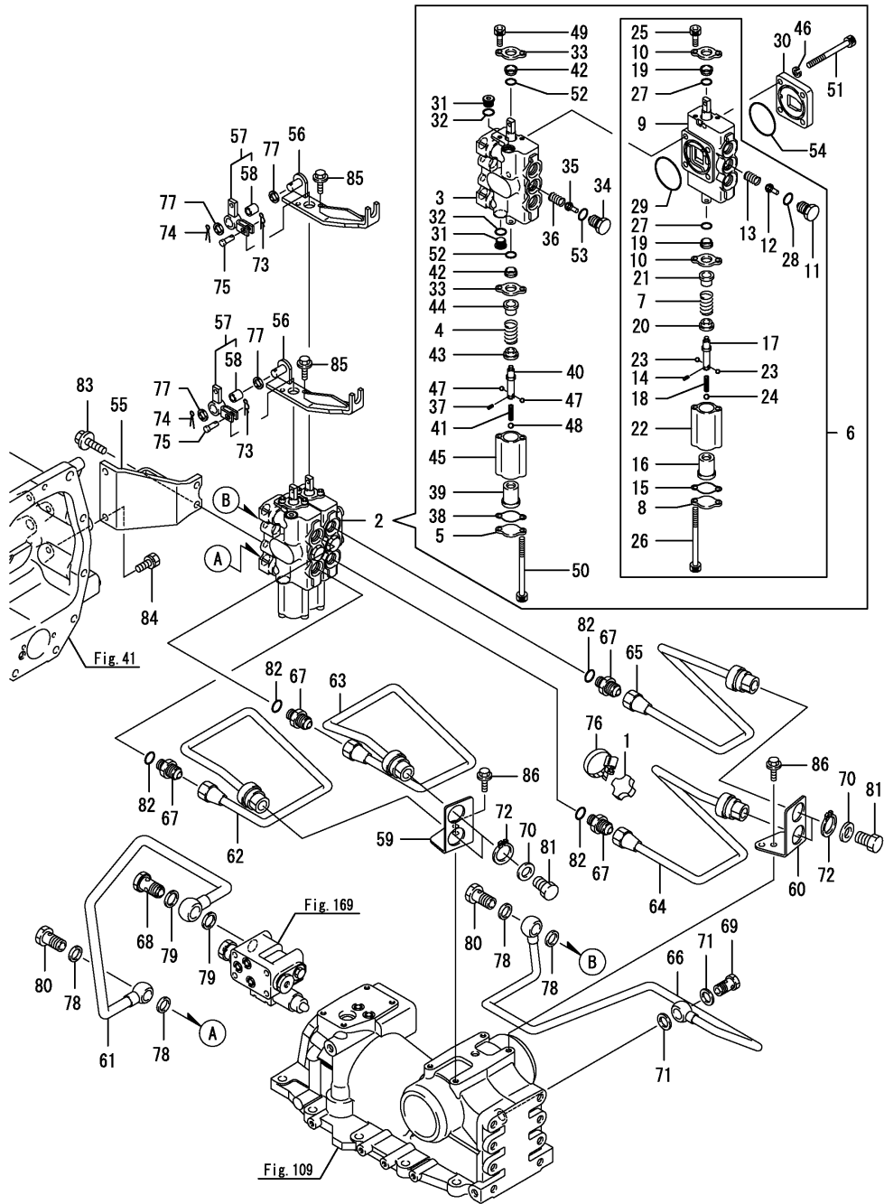
Fig.117. 보조컨트롤밸브
