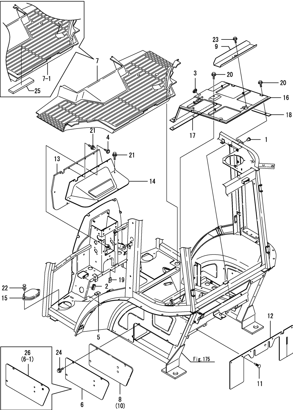
Fig.177. 캐빈
