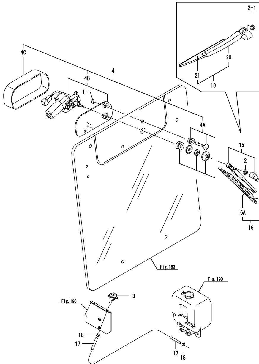
Fig.192. 후방와이퍼
