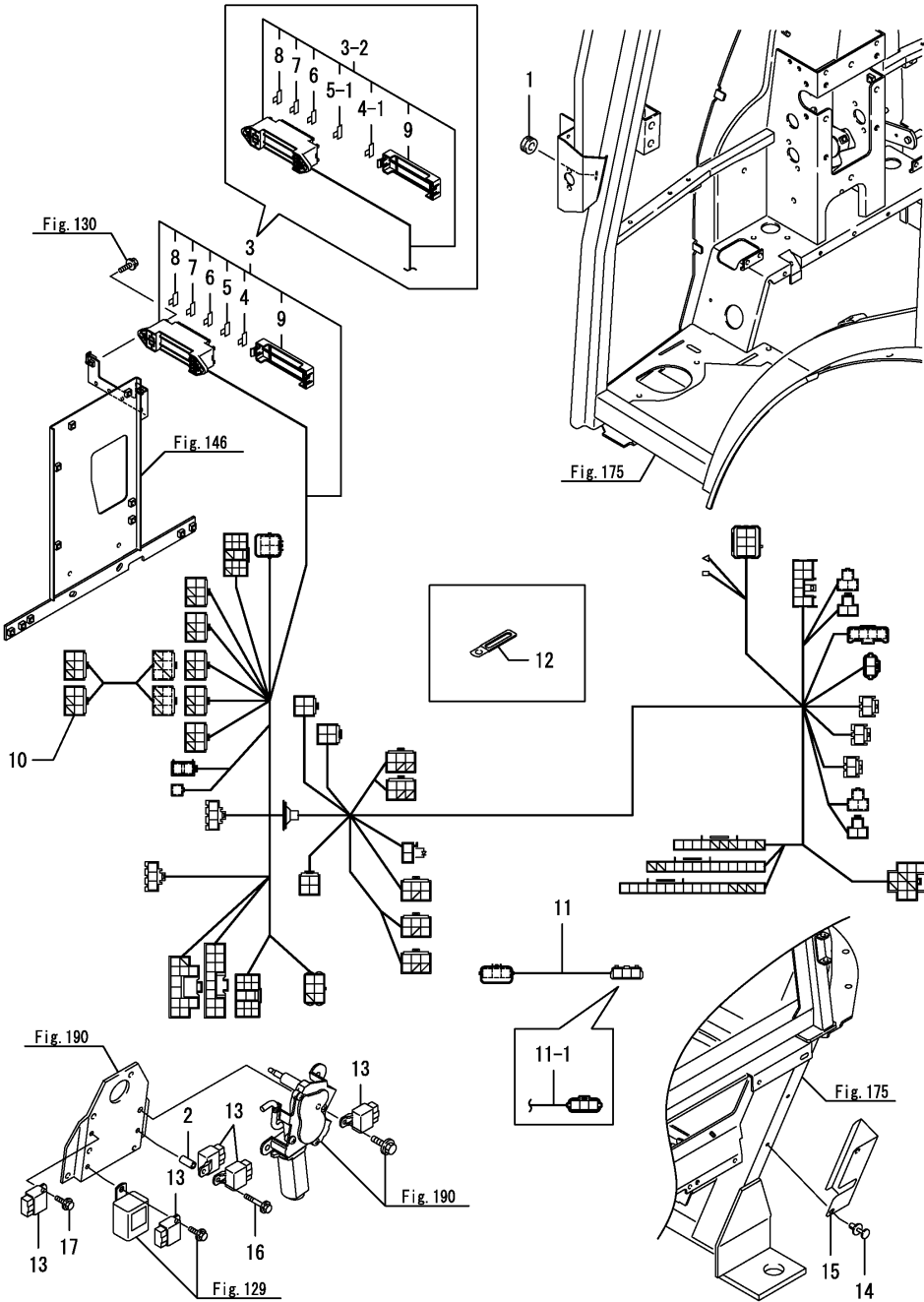
Fig.132. 배선(캐빈)
