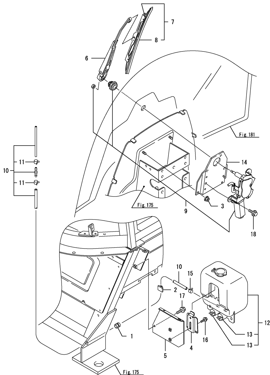
Fig.190. 전방와이퍼
