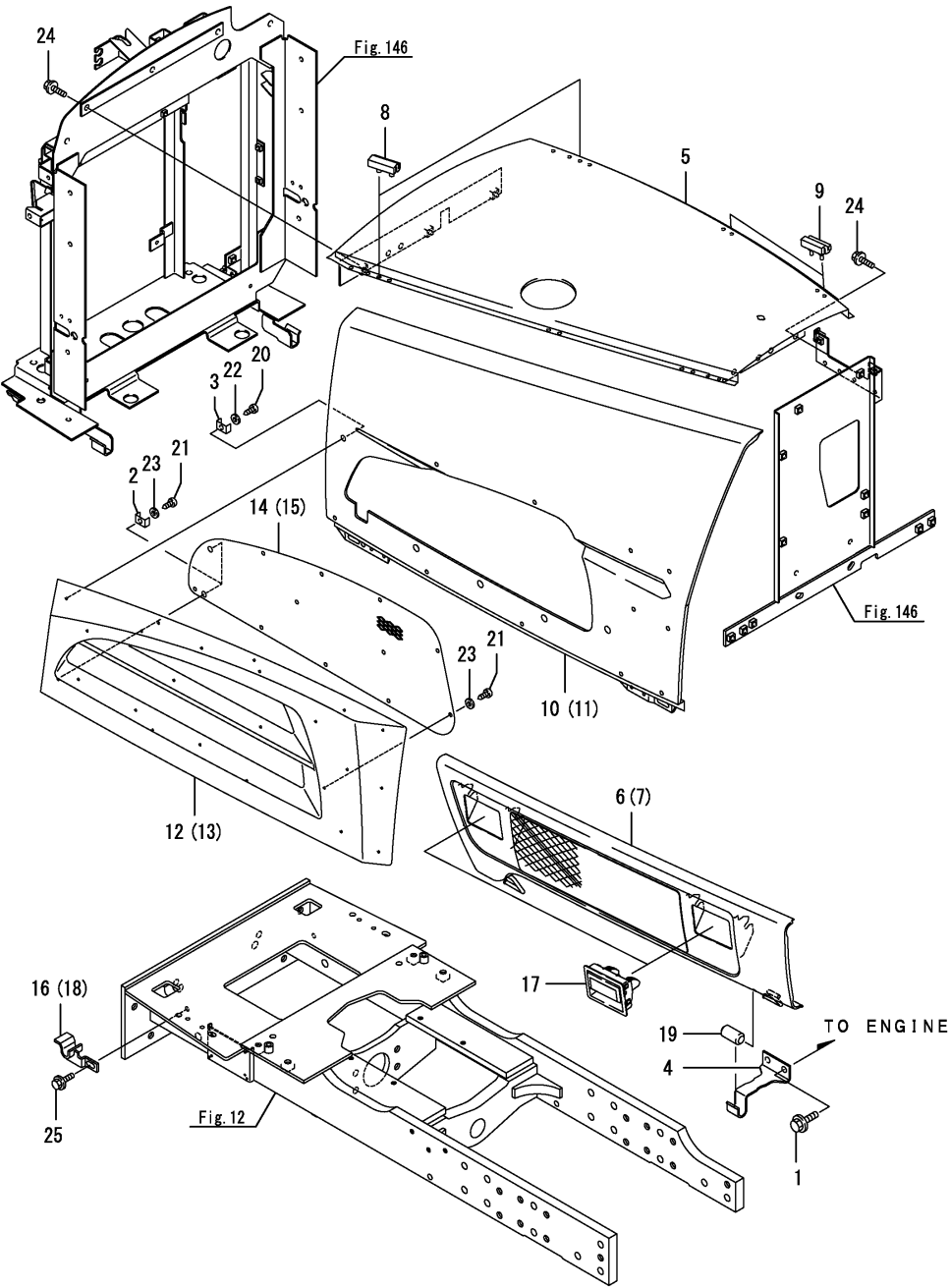
Fig.147. 본네트
