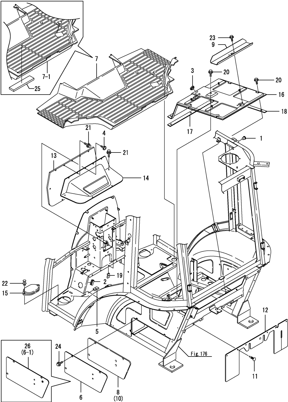
Fig.178. 캐빈
