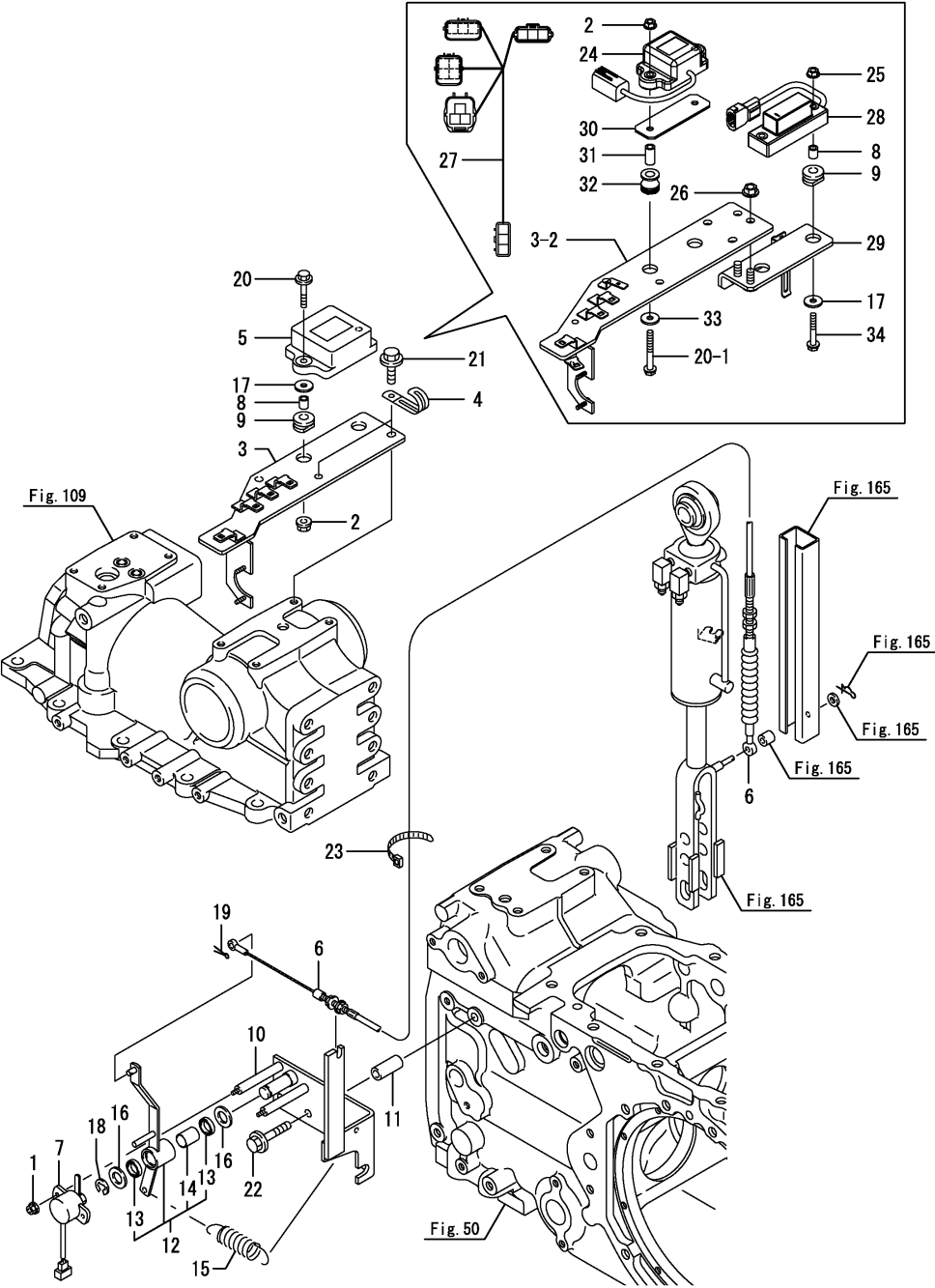
Fig.171. 수평 제어센서
