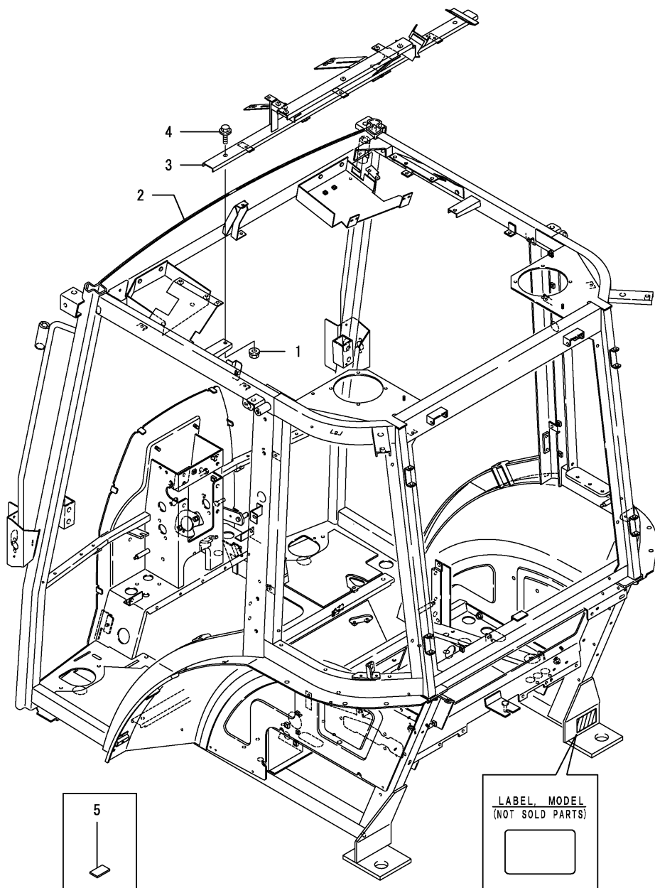
Fig.176. 캐빈프레임
