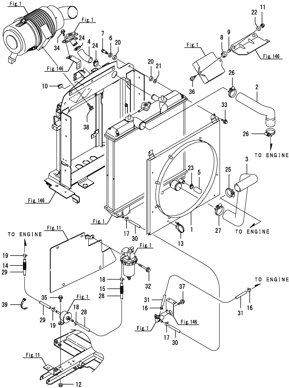
Fig.3. 엔진악세사리
