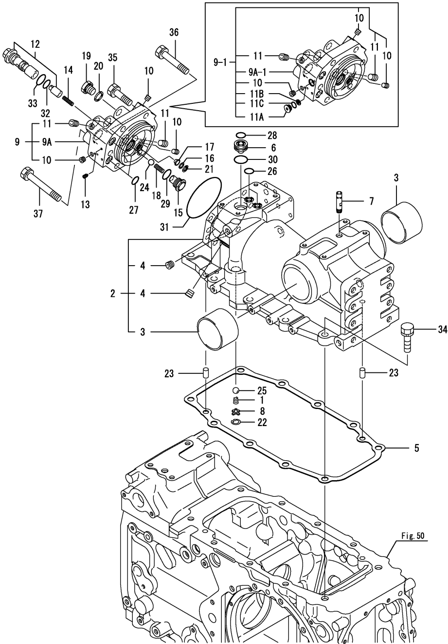
Fig.110. 유압실린더케이스
