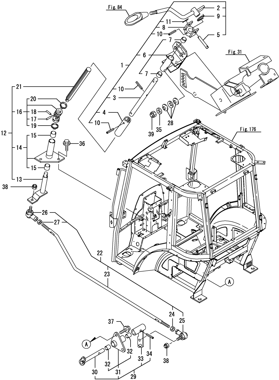
Fig.76. 리버서레버
