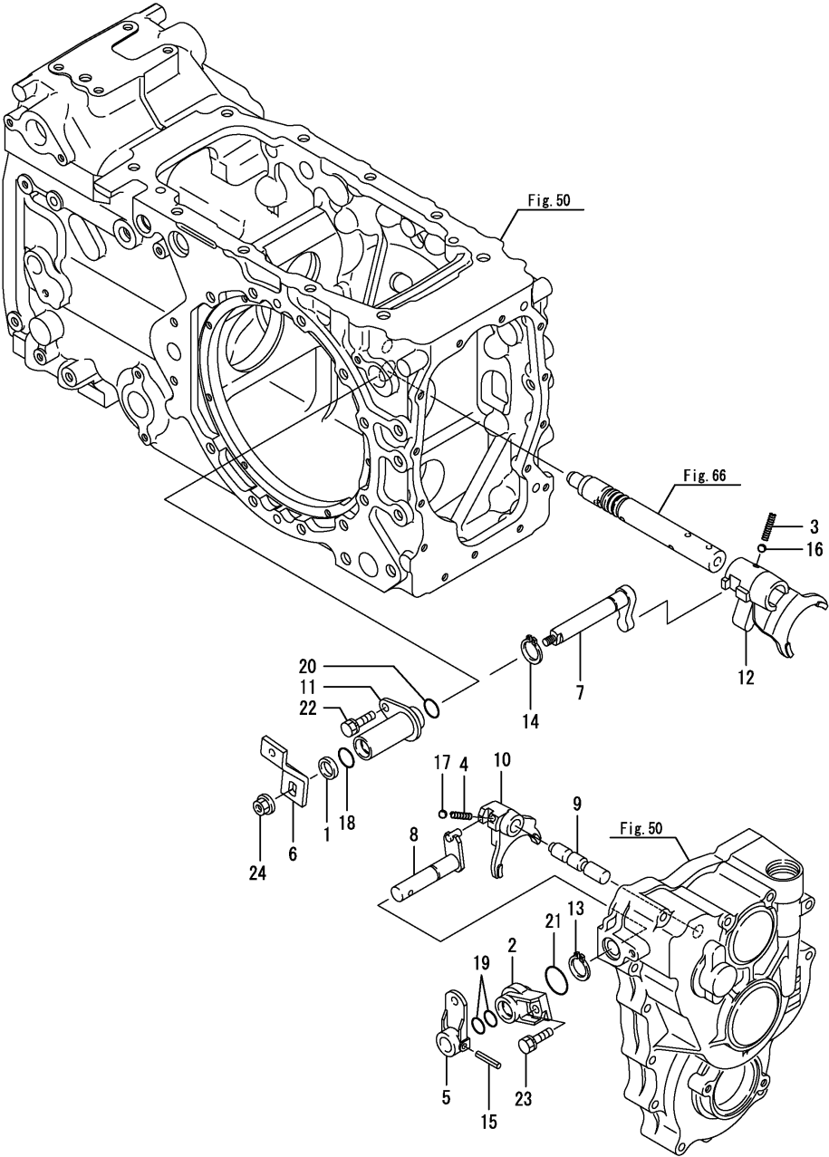
Fig.83. P.T.O. 변속
