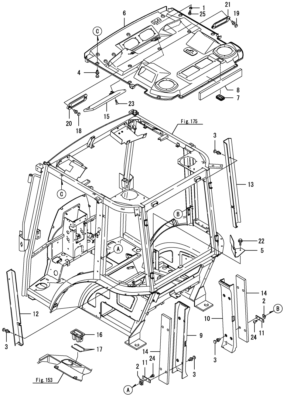
Fig.184. 인테리어
