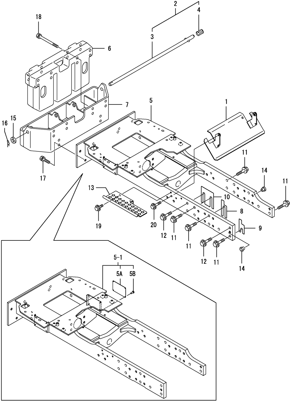
Fig.13. 프론트브라켓
