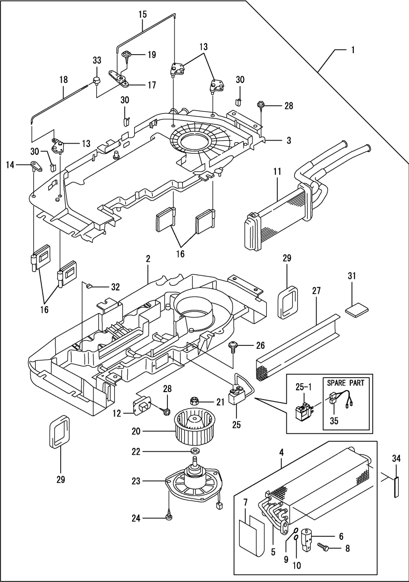
Fig.196. 에어컨(유닛) (내부 부품)
