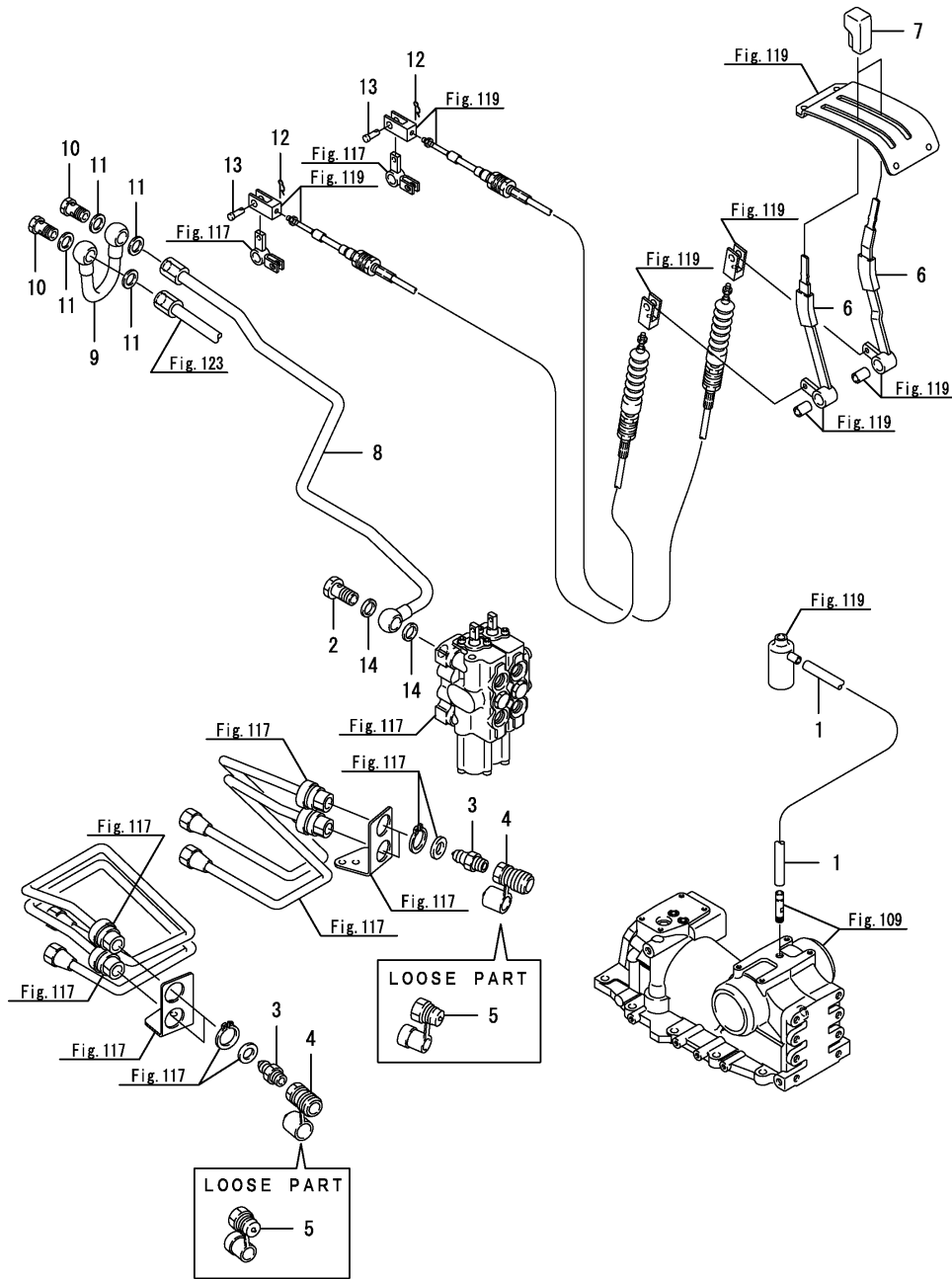
Fig.118. S.C.V.컨트롤
