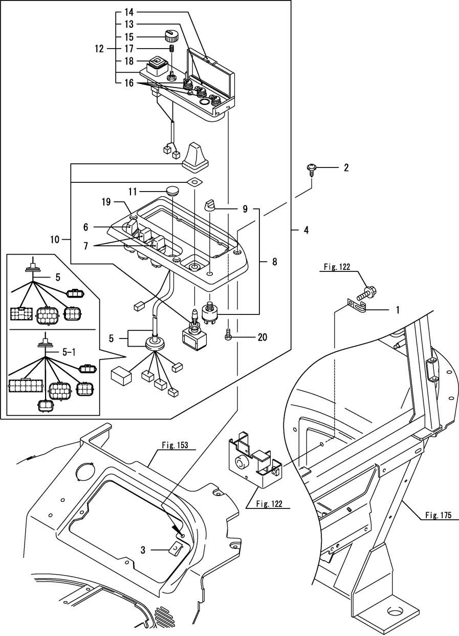
OCNP4-M98801 히치부 Fig.172. 컨트롤박스
