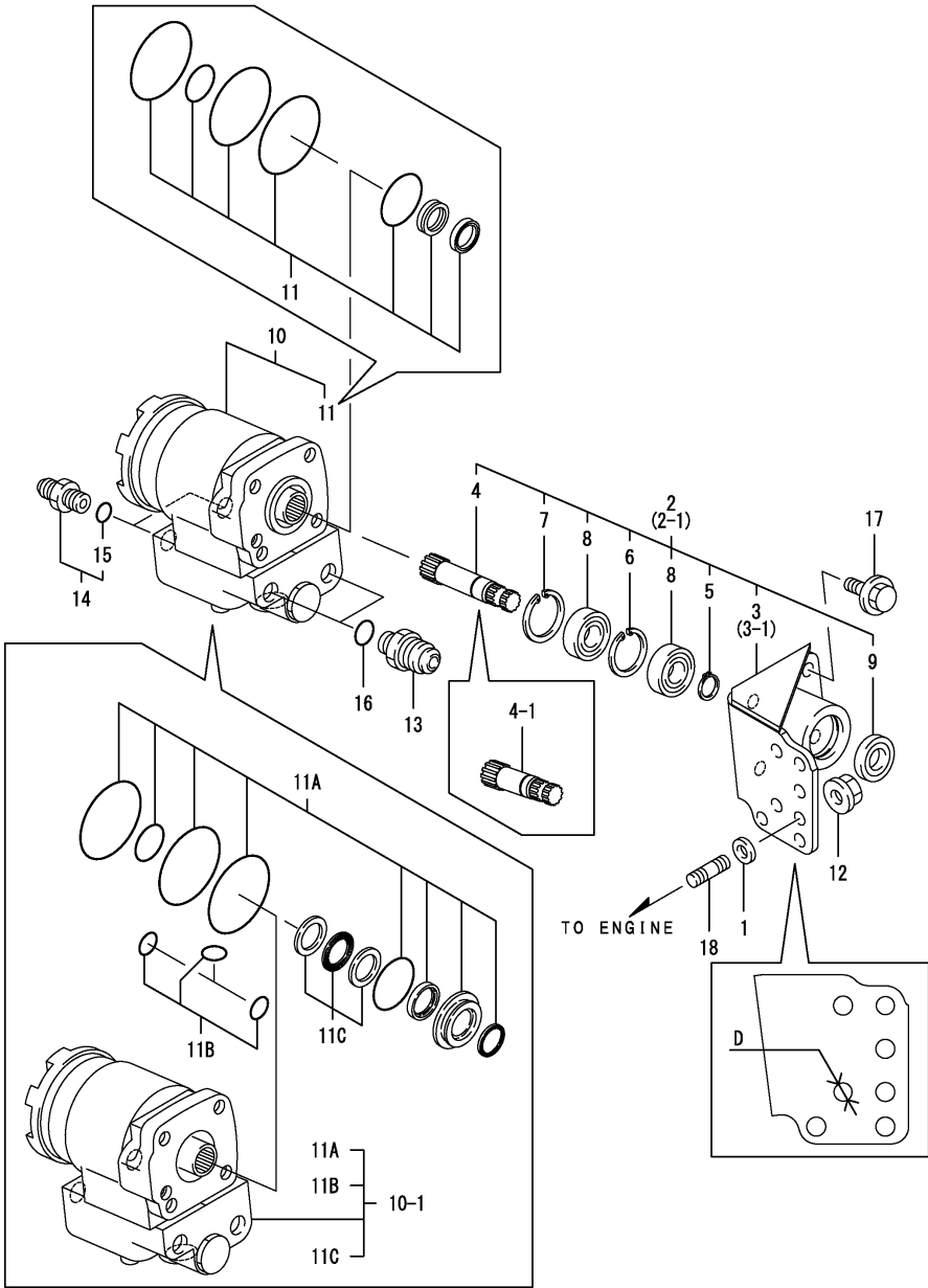
Fig.36. P.S.T.밸브
