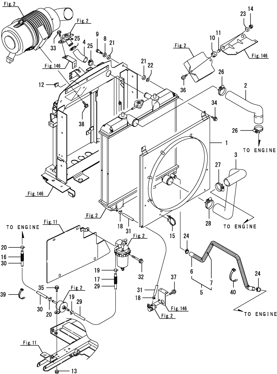
Fig.4. 엔진악세사리
