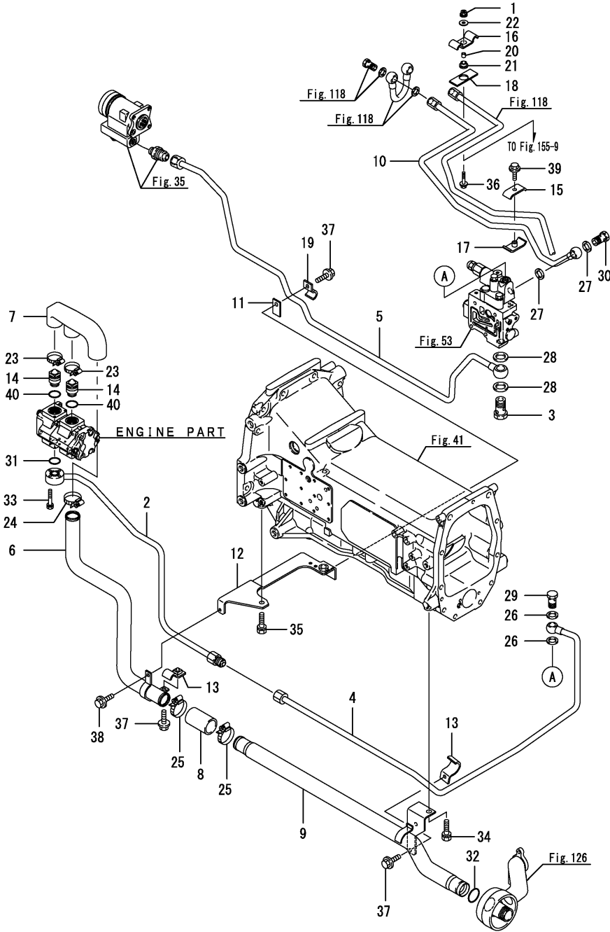
Fig.123. 유압배관
