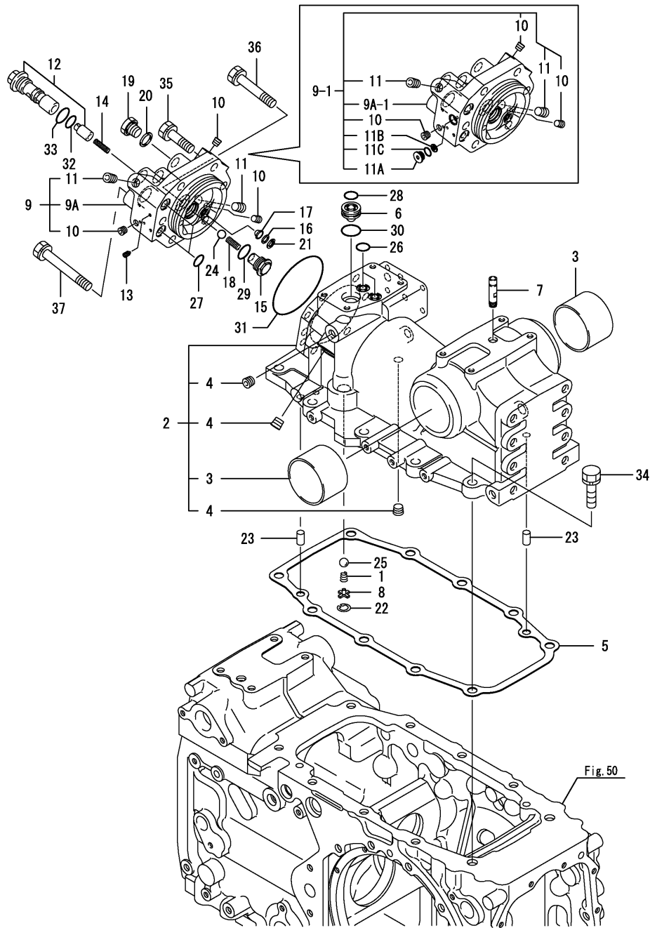
Fig.109. 유압실린더케이스
