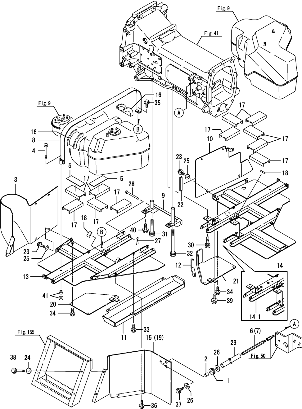
Fig.11. 탱크커버
