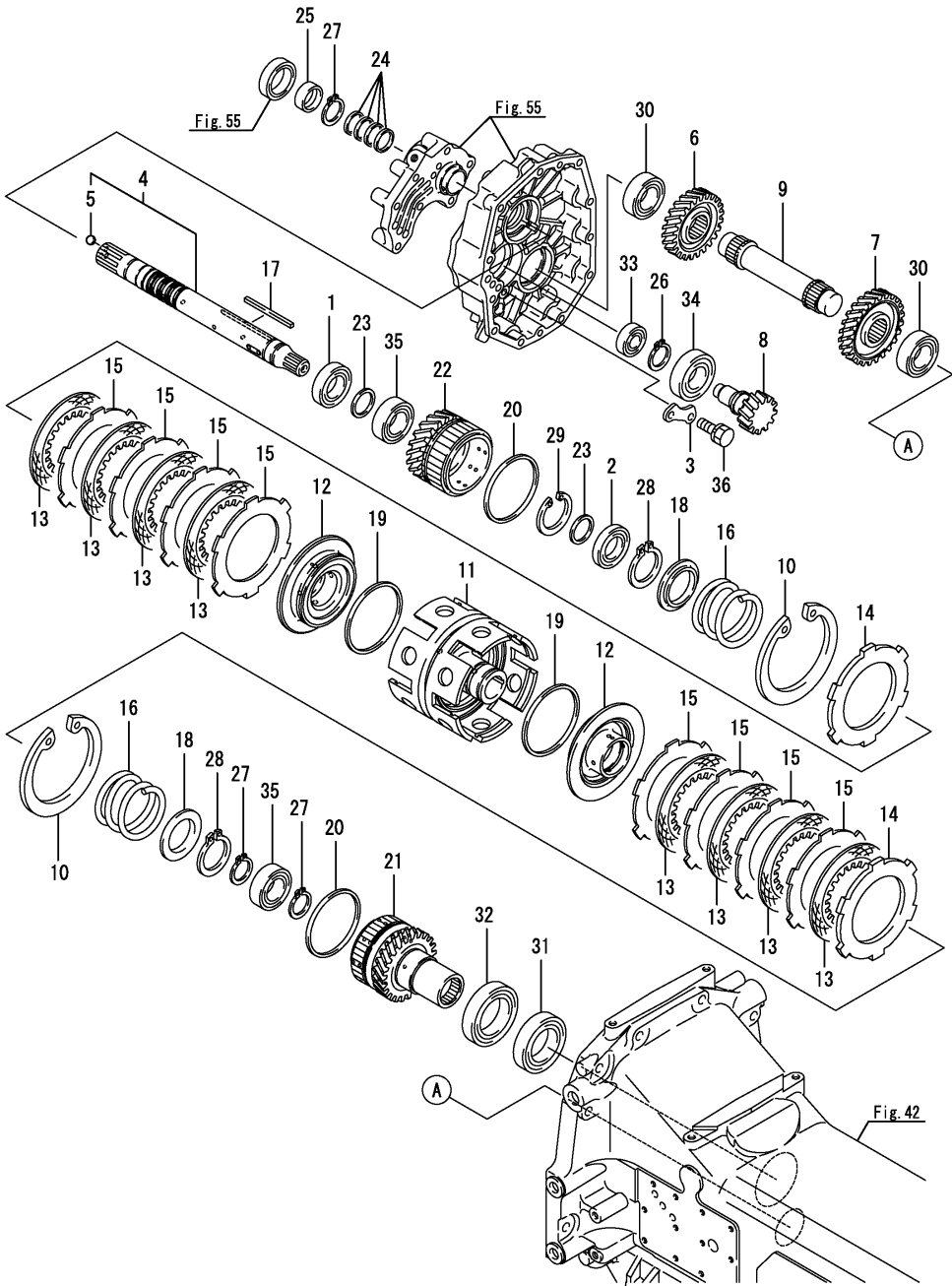
Fig.62. 파워리버서
