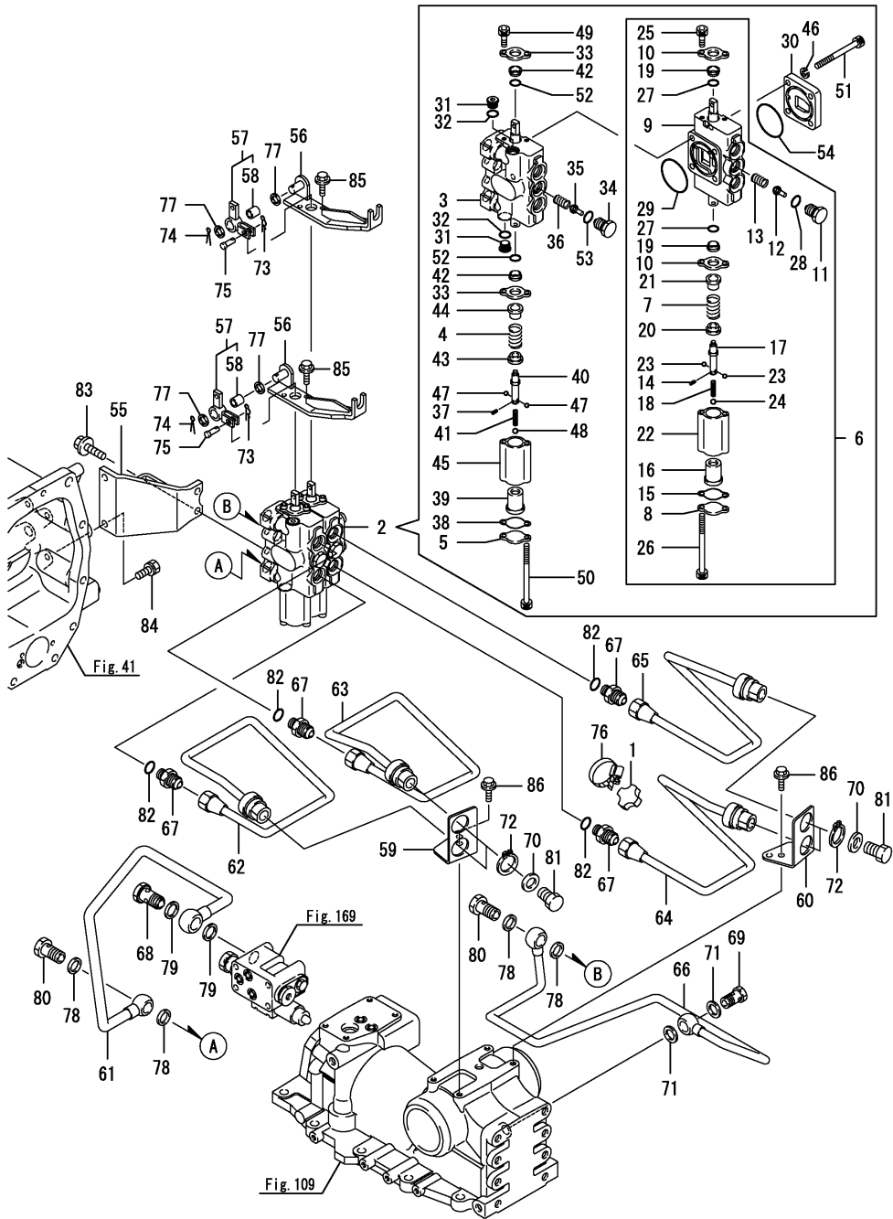
Fig.117. 보조컨트롤밸브
