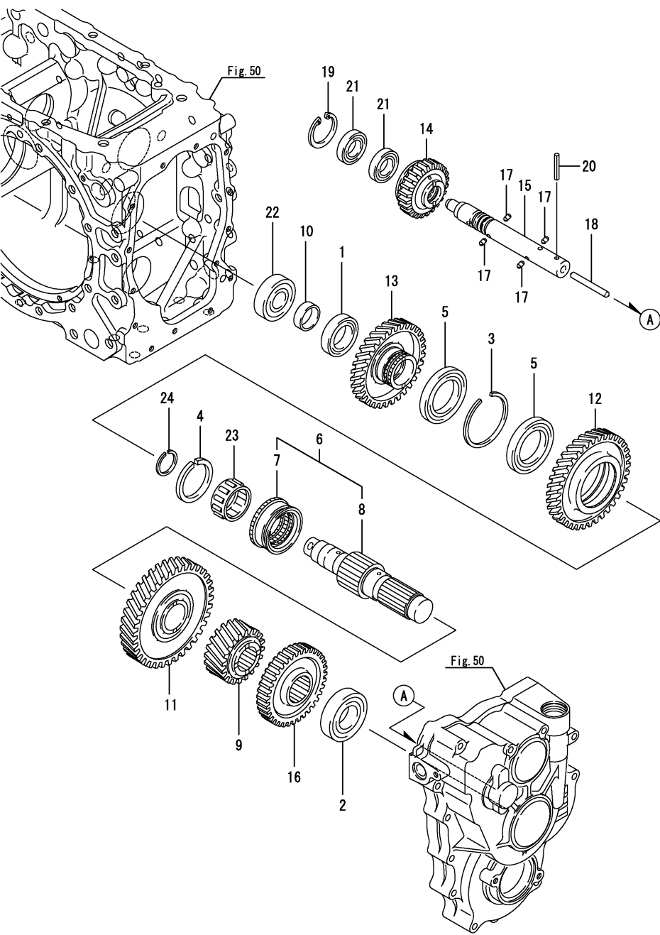
Fig.66. P.T.O. 피구동축
