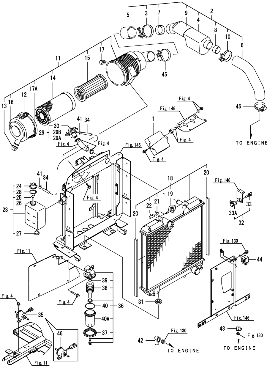
Fig.2. 엔진관련
