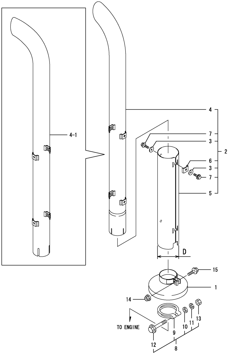
Fig.8. 배기구
