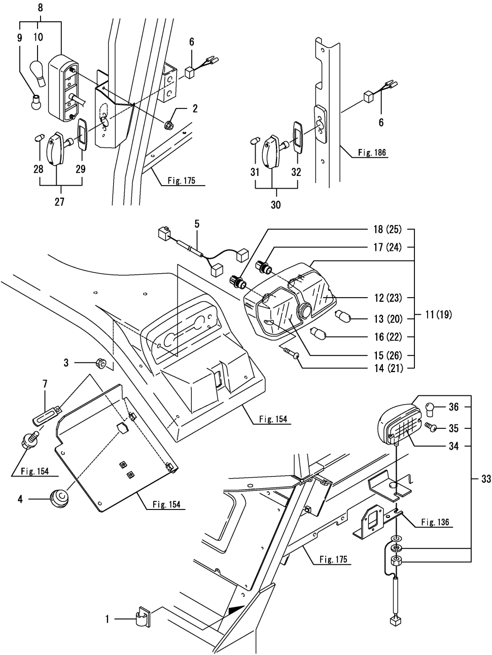
Fig.141. 램프
