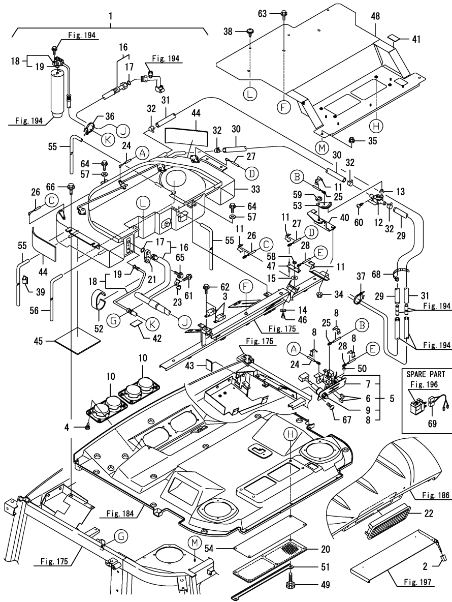
Fig.195. 에어컨
