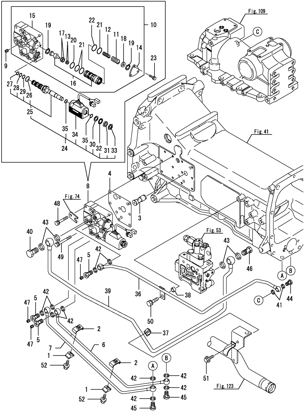
Fig.87. 프론트시프트
