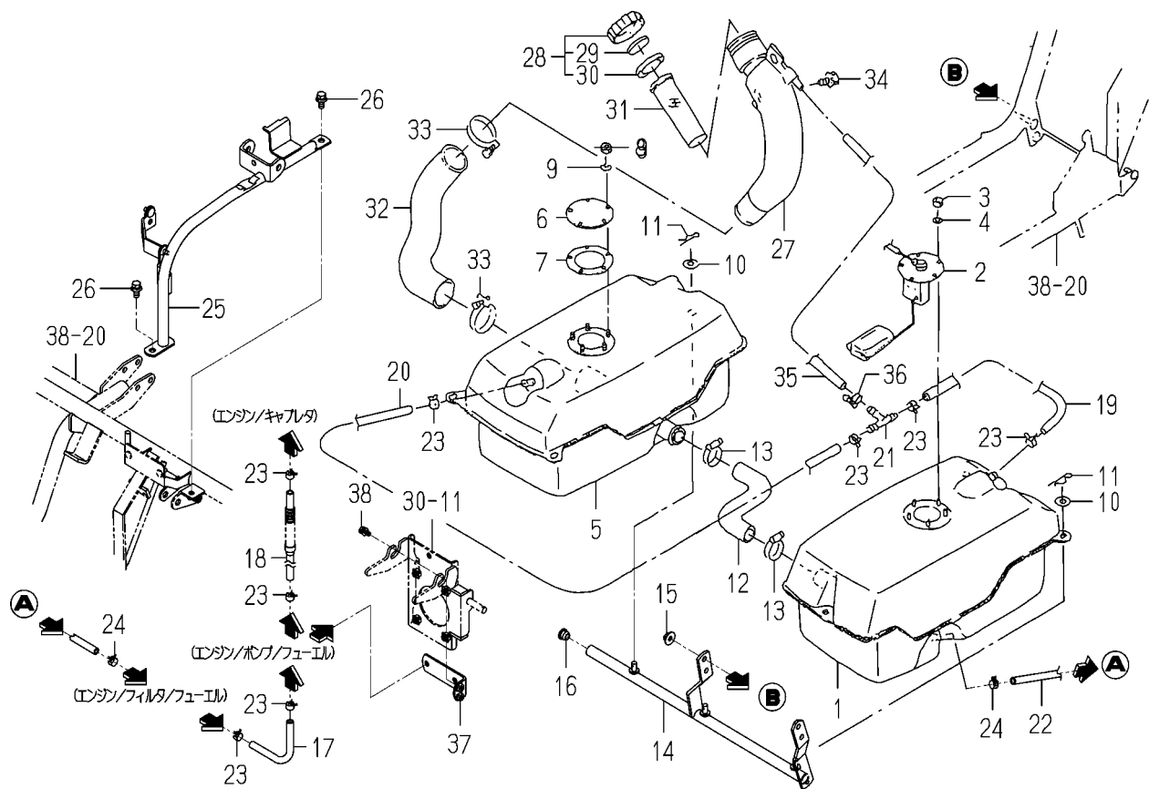
FIG. 4 ヒューエルタンク関係
