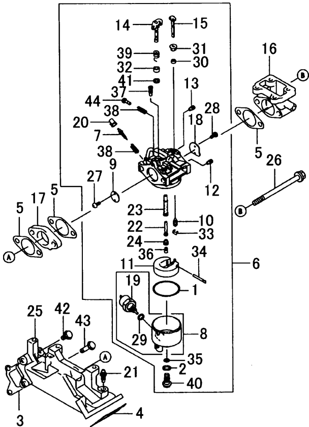
FIG. 8 キャブレタ
