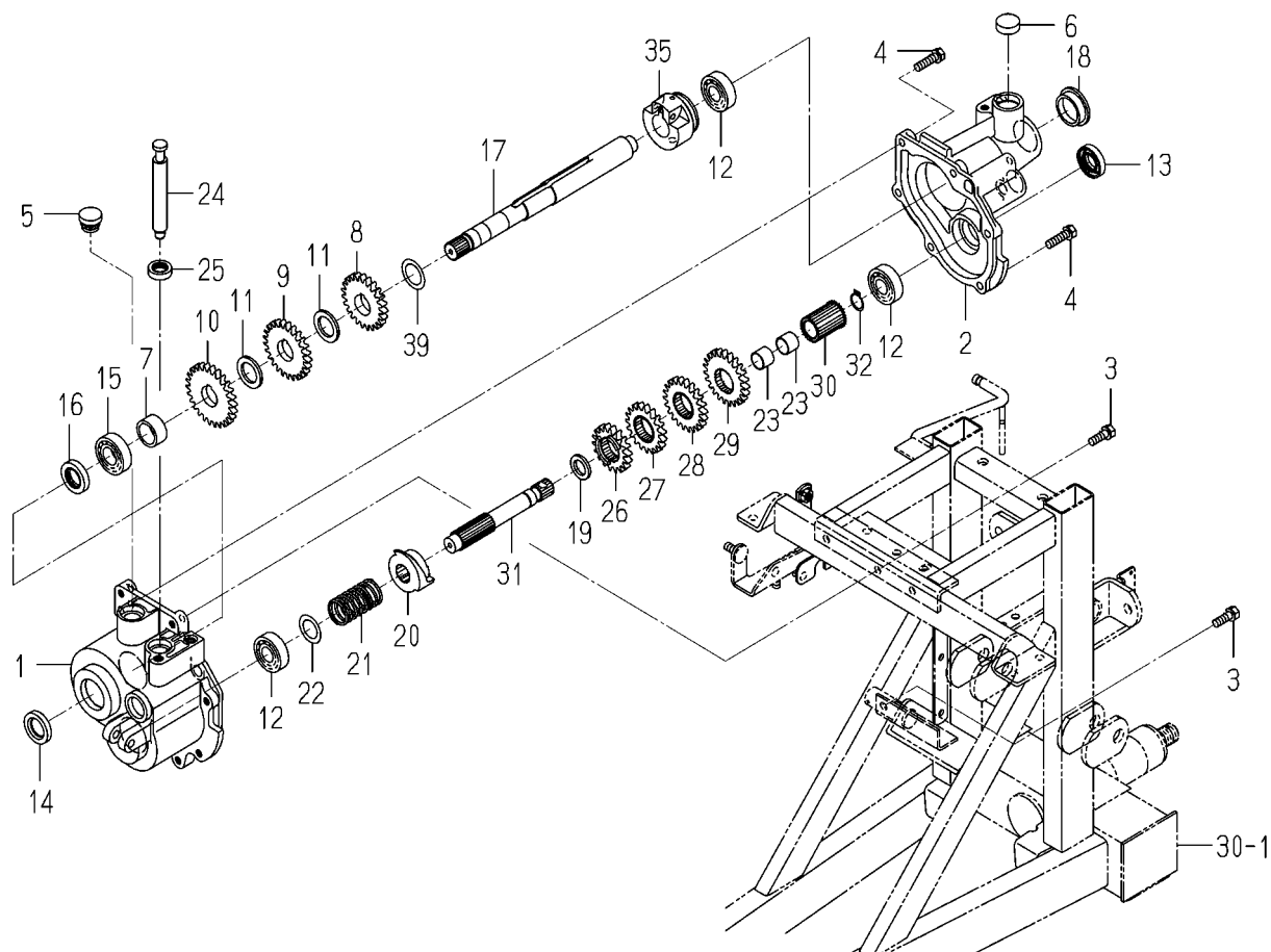
FIG. 46 ウエツケドウケース関係(図1/2)
