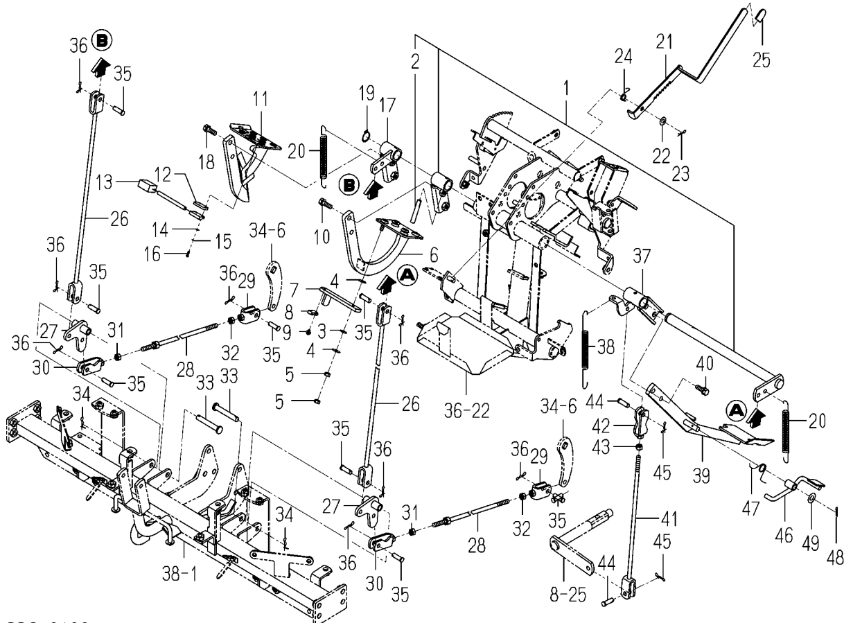
FIG. 37 ペダル(ブレーキ/クラッチ)関係
