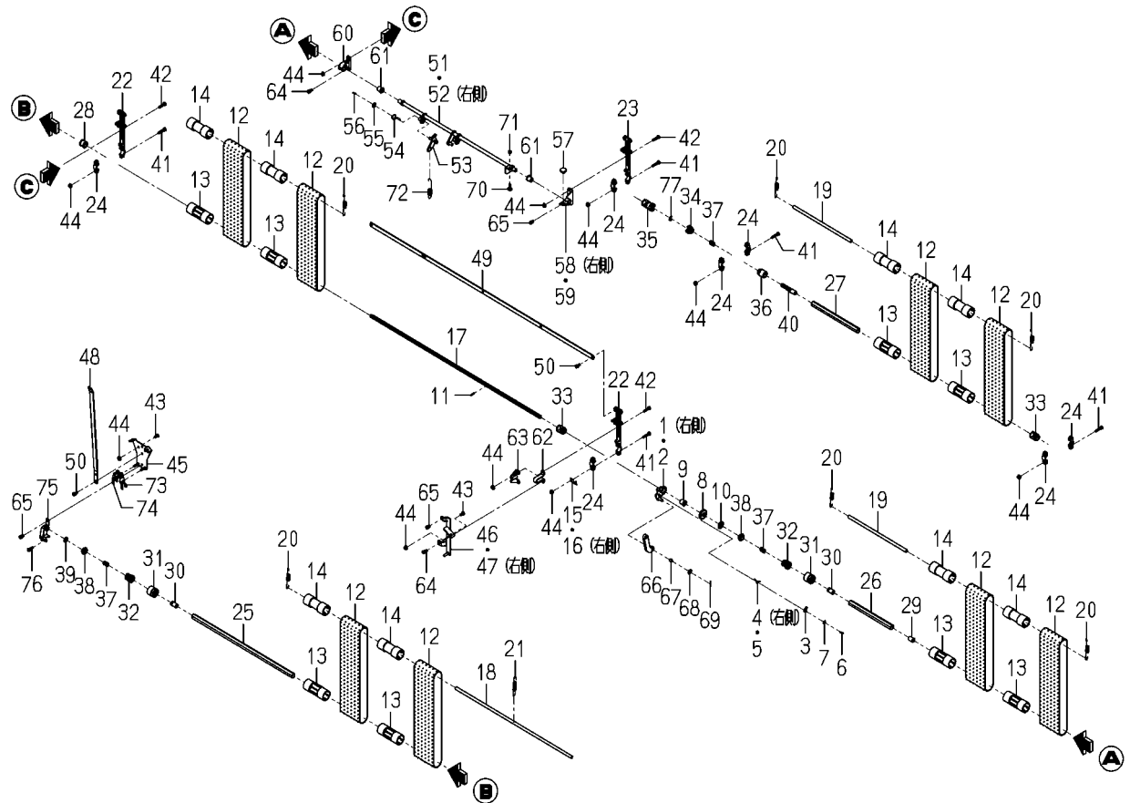
FIG.105 ナエオクリ関係
