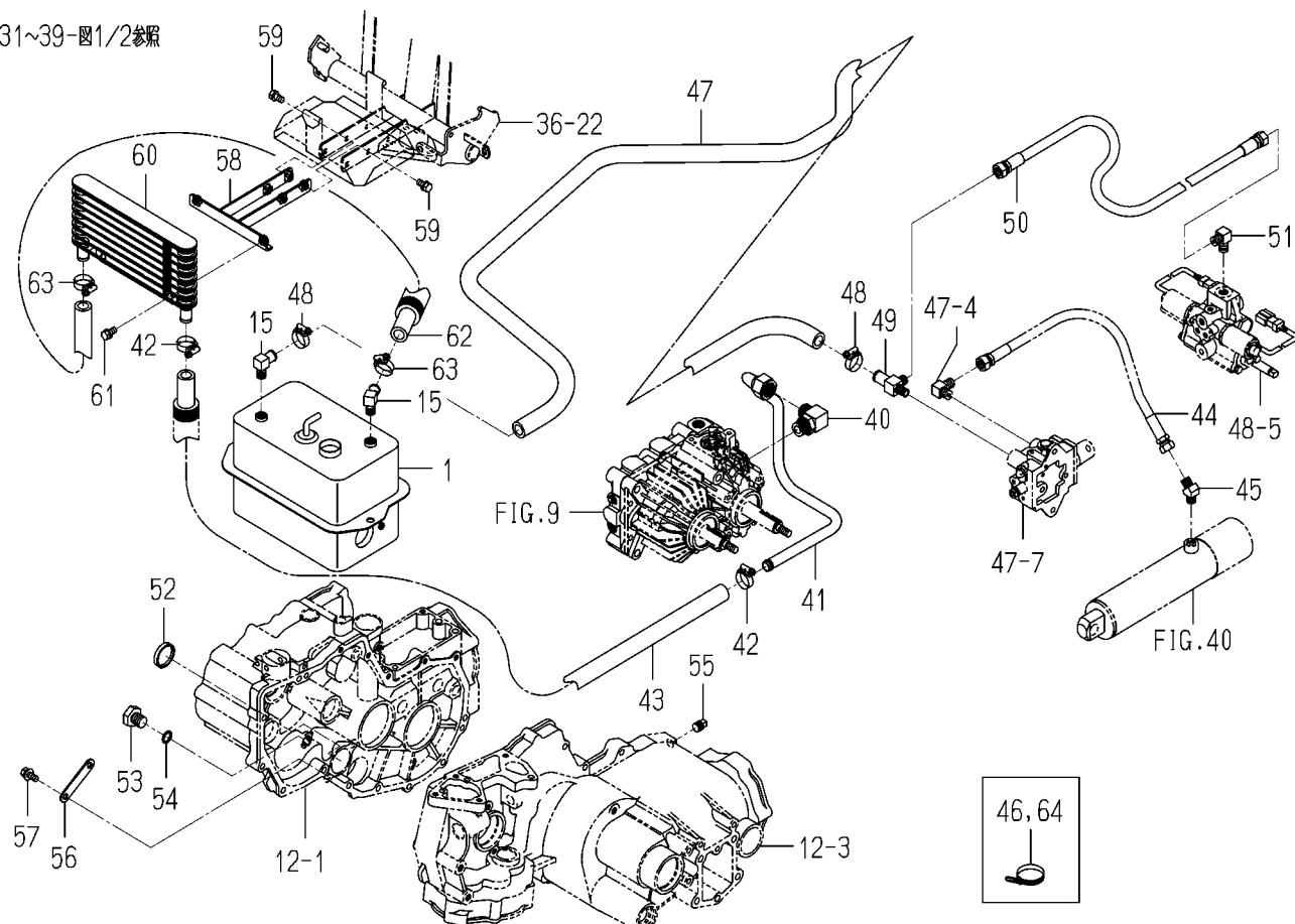
FIG. 41 ハイカン関係(図2/2)
