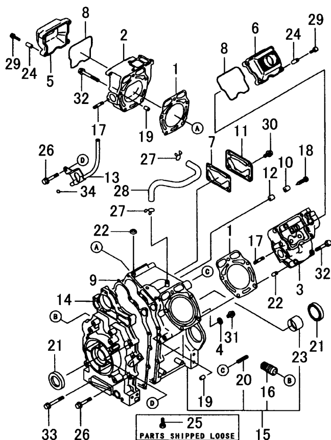
FIG. 1 シリンダ／クランクケース
