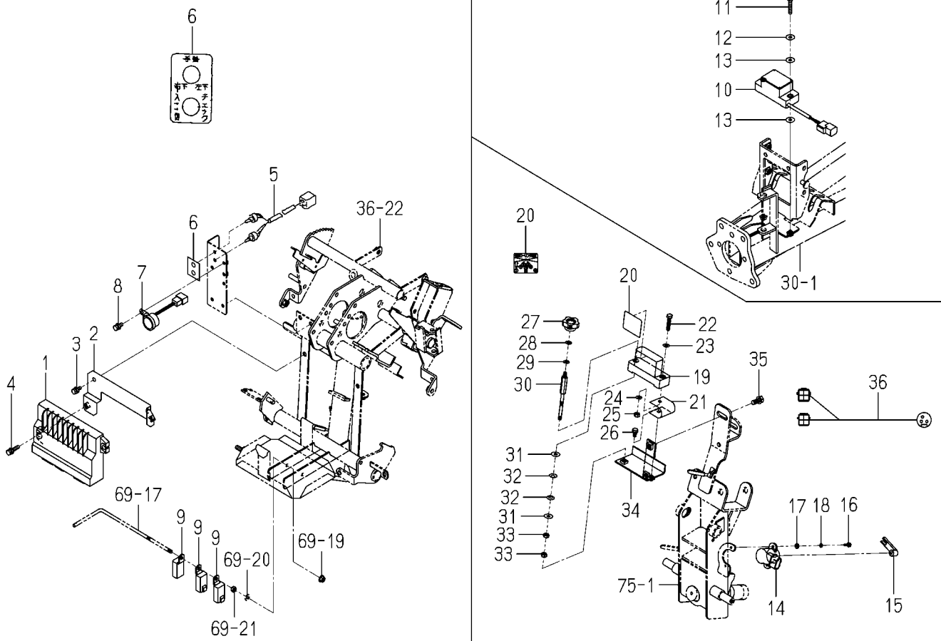
FIG. 73 マイコン関係
