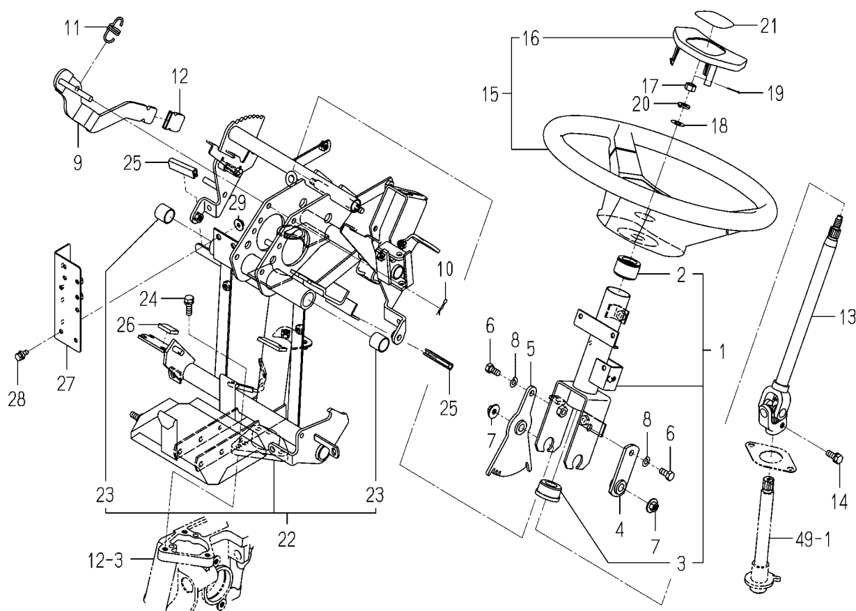
FIG. 36 ステアリング関係
