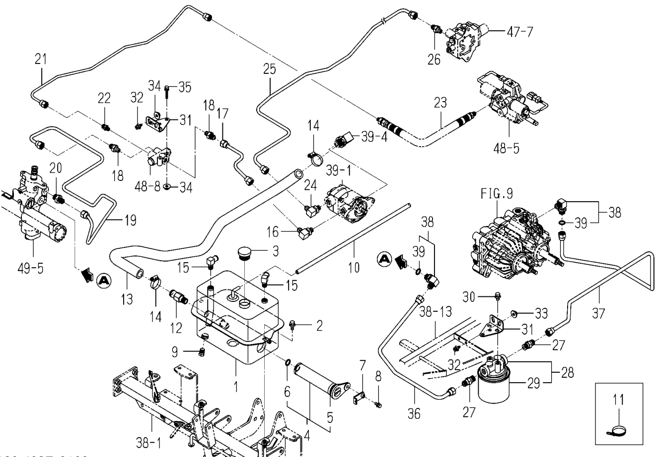
FIG. 41 ハイカン関係(図1/2)
