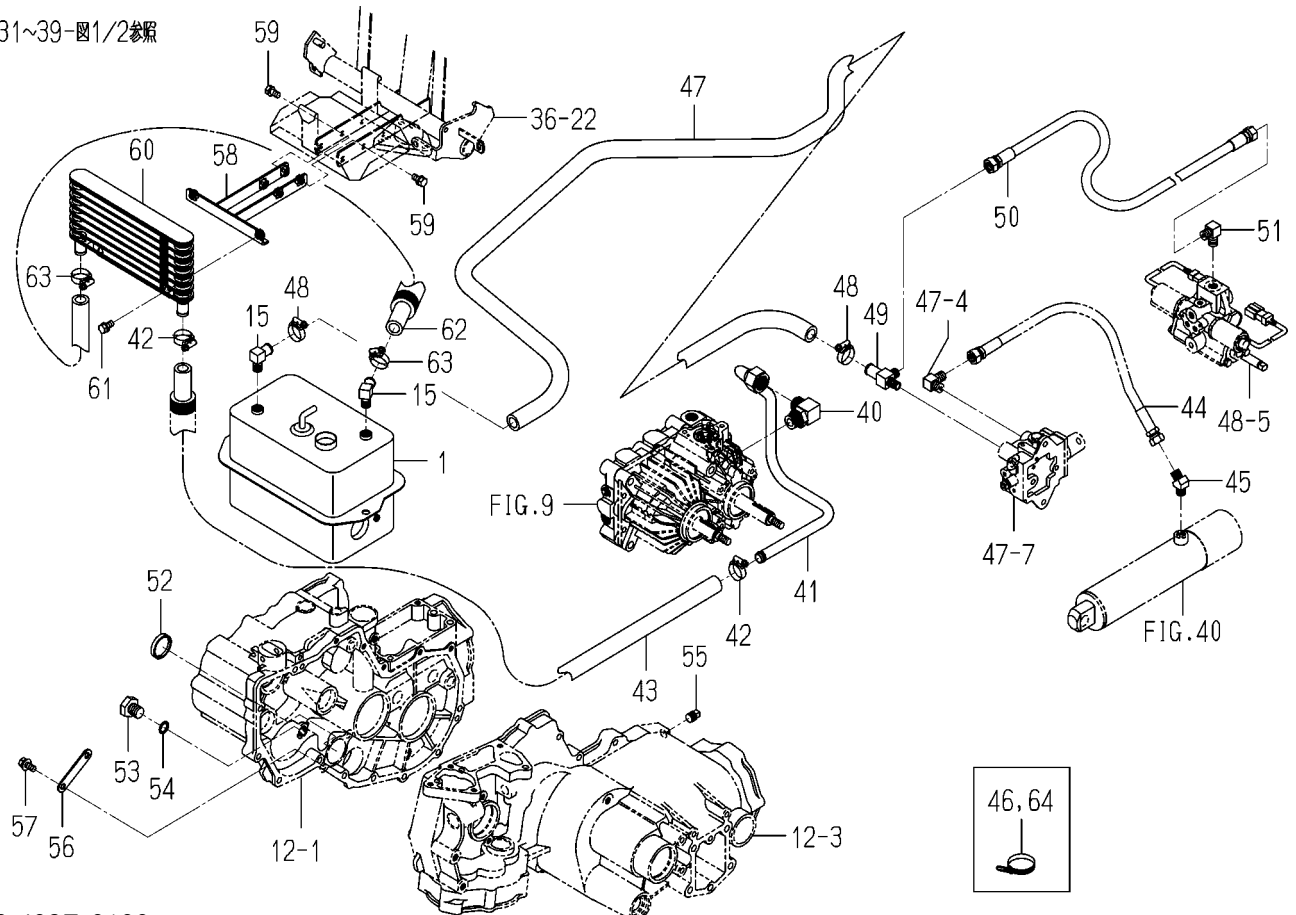
FIG. 41 ハイカン関係(図2/2)
