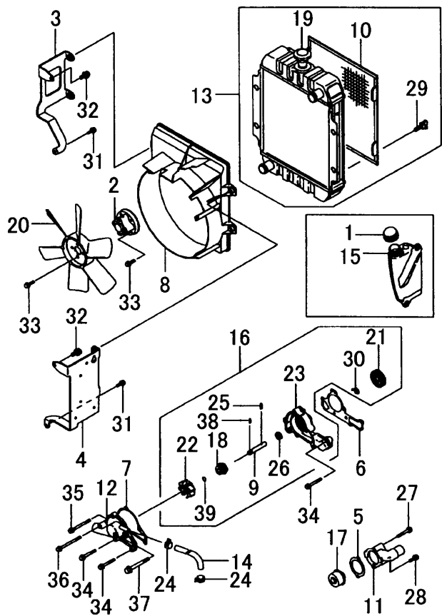
FIG. 5 レイキヤクソウチ
