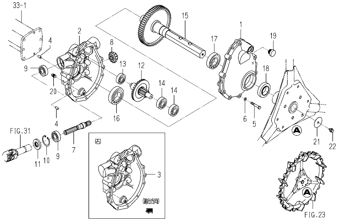
FIG. 35 ケース(リヤ)関係
