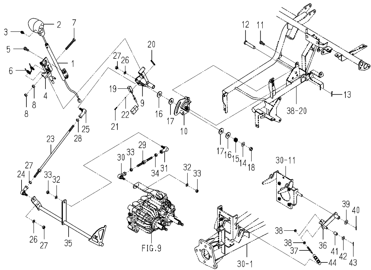
FIG. 7 レバー(HST)関係
