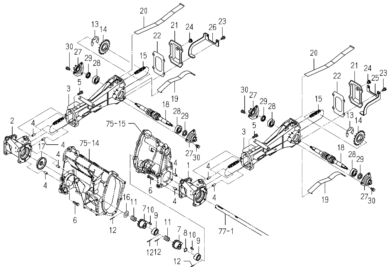
FIG. 81 ウエコミカンジク関係
