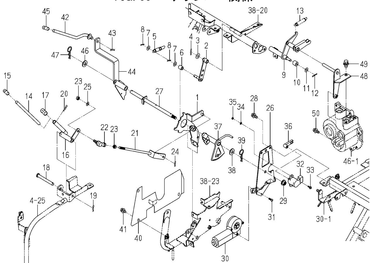
FIG. 65 ユアツレバー関係
