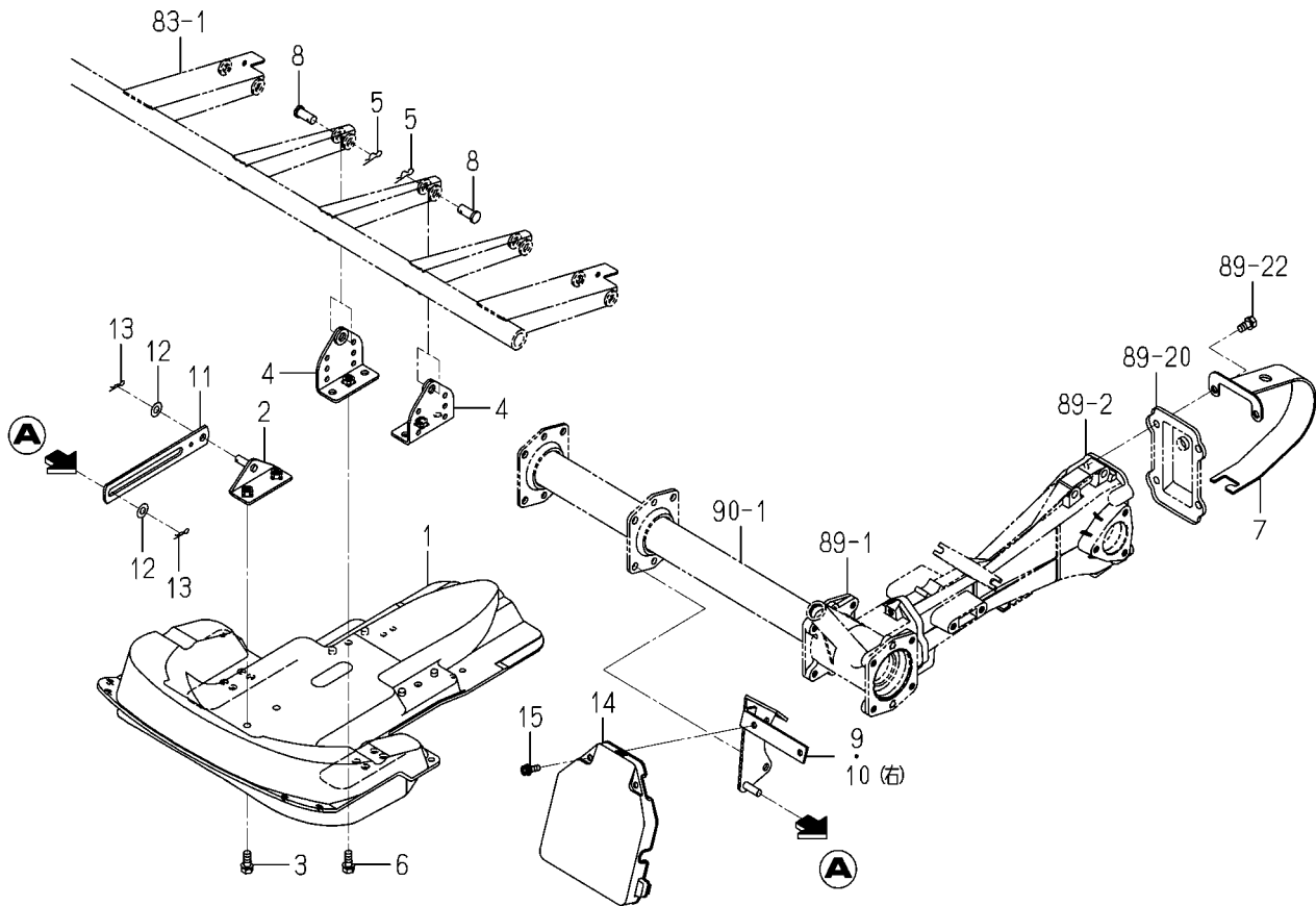
FIG. 97 フロート(サイド)関係
