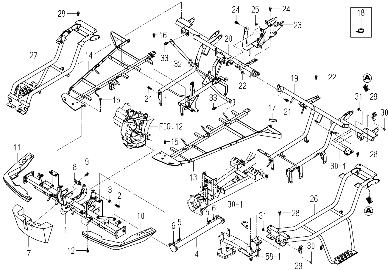
FIG. 38 バンパ、サイドフレーム関係
