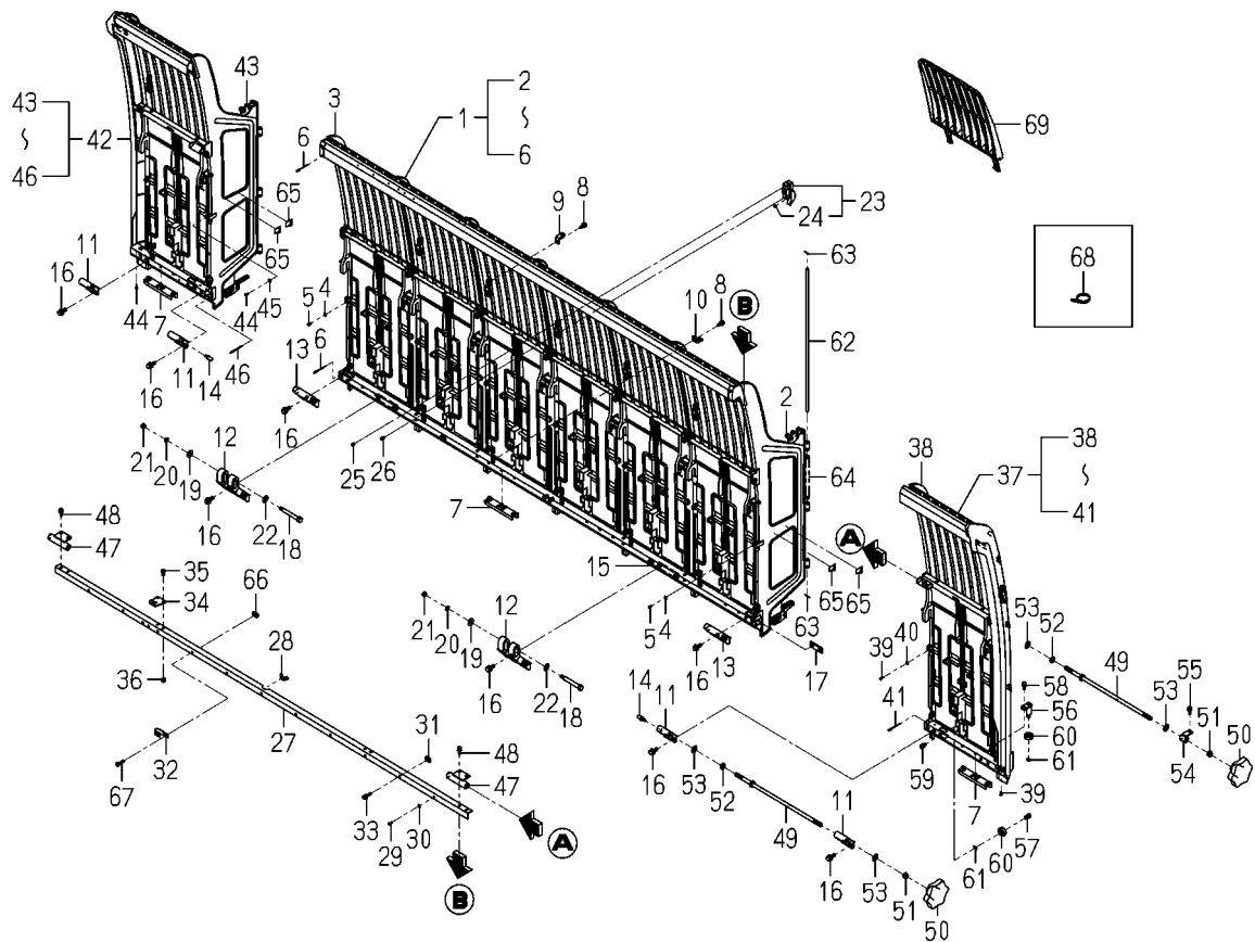
FIG.101 ナエタンク関係
