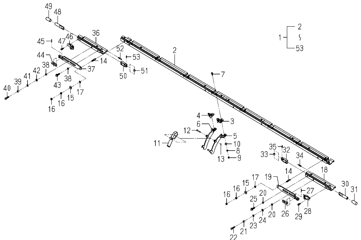
FIG.114 マエイタ(コウカン)SET(オプション)
