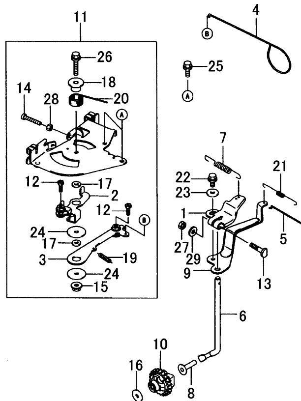
FIG. 7 コントロールソウチ
