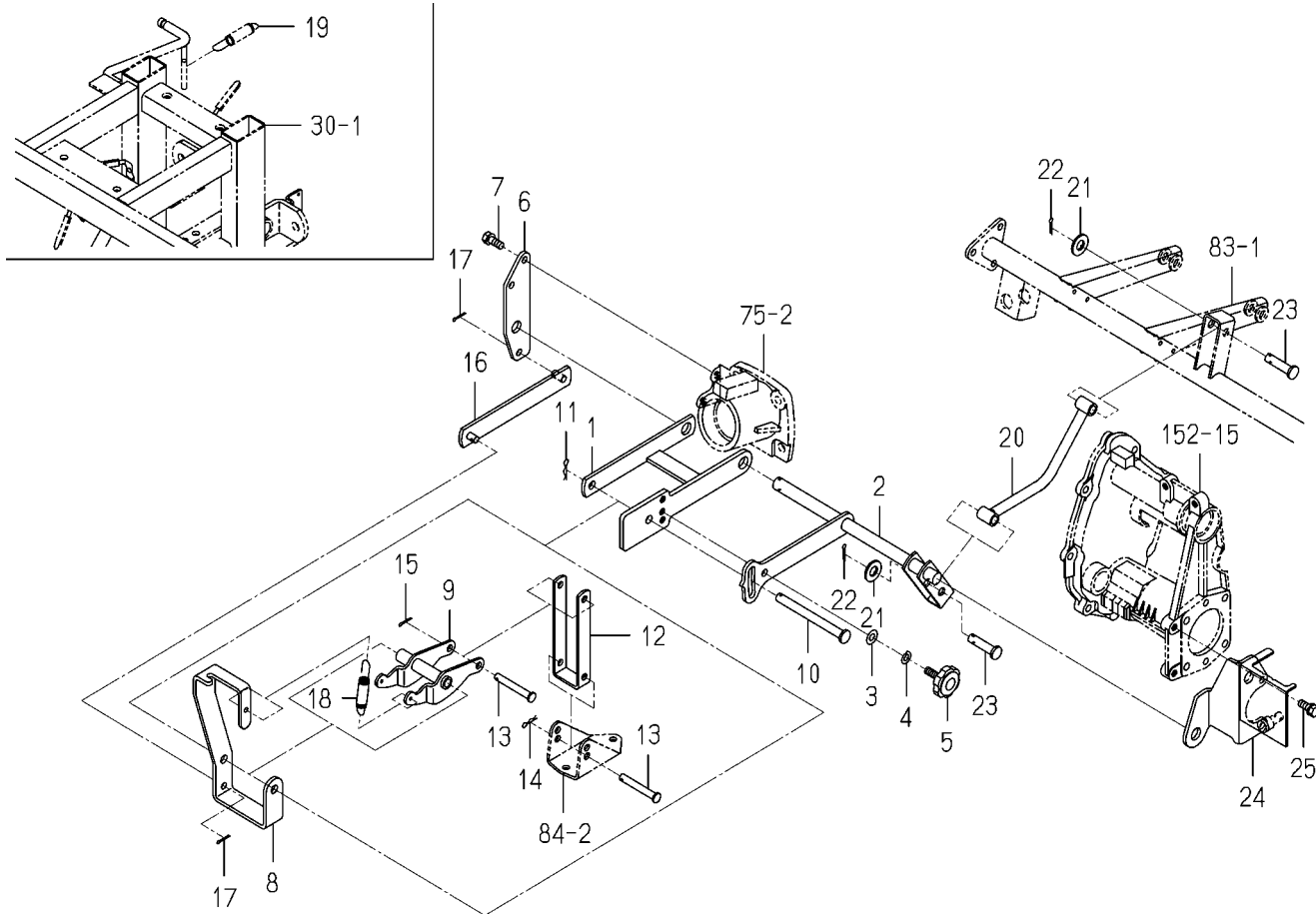
FIG. 85 フロートリンク関係
