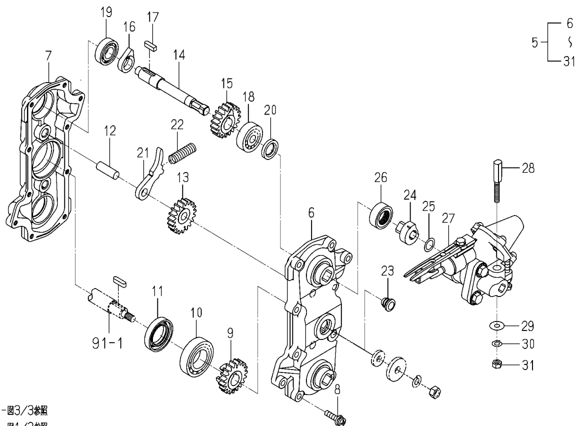
FIG.108 フゾクヒン(図2/3)
