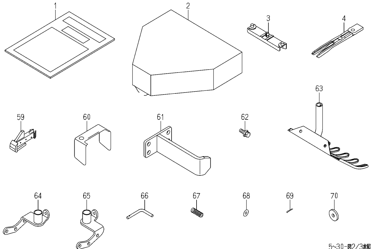
FIG.108 フゾクヒン(図1/3)
