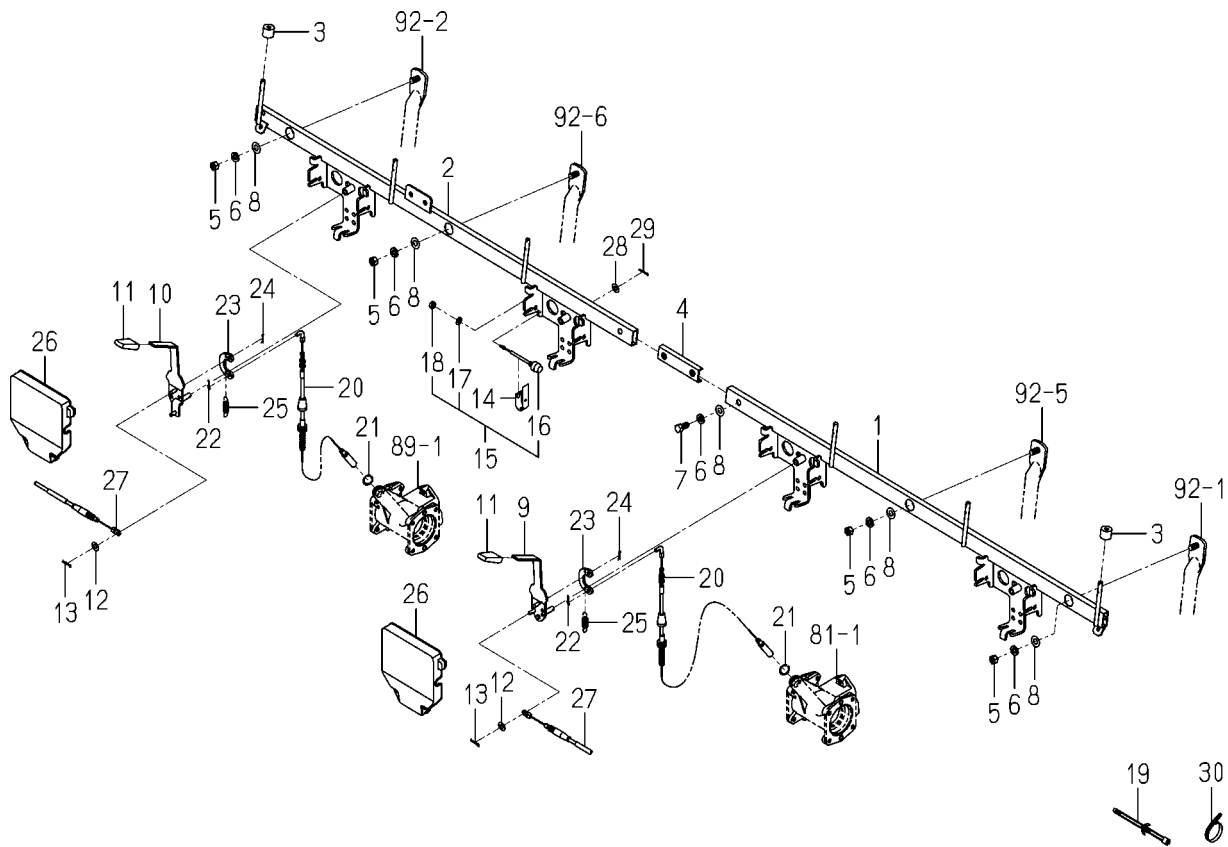
FIG. 93 ステー(アゼクラッチ)関係
