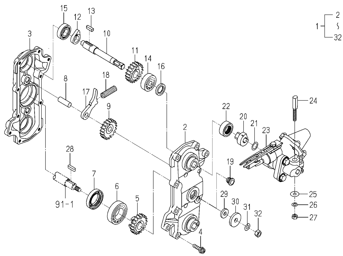
FIG. 99 ロータリウエコミカン(LH)関係
