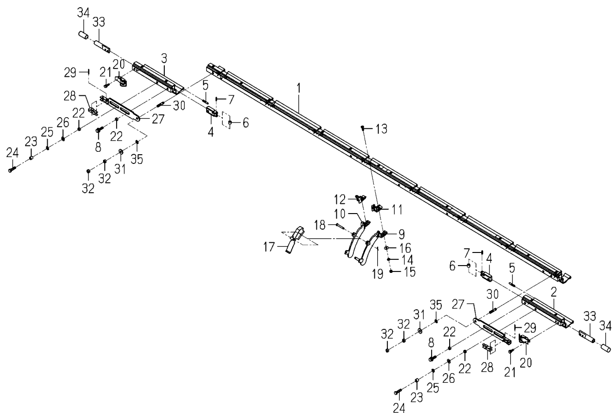
FIG.103 マエイタ関係
