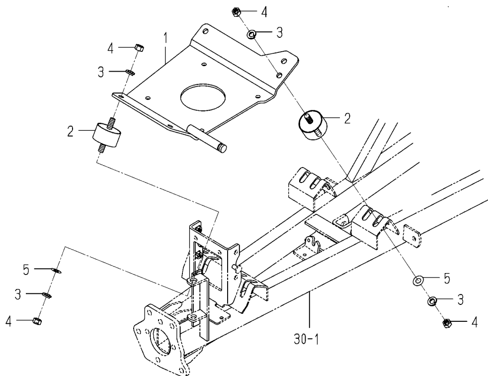
FIG. 2 エンジントリツケ関係
