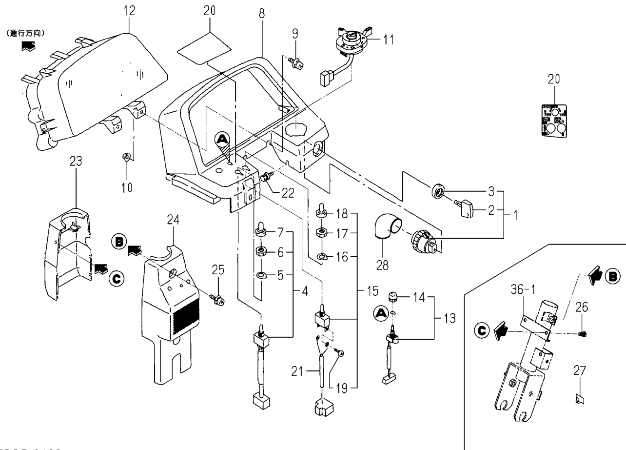
FIG. 68 メータパネル関係
