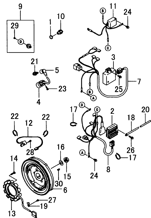
FIG. 6 デンソウヒン
