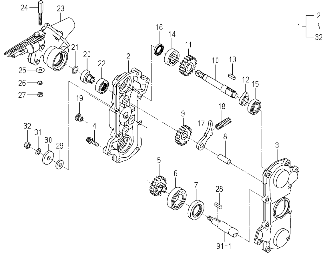
FIG.100 ロータリウエコミカン(RH)関係
